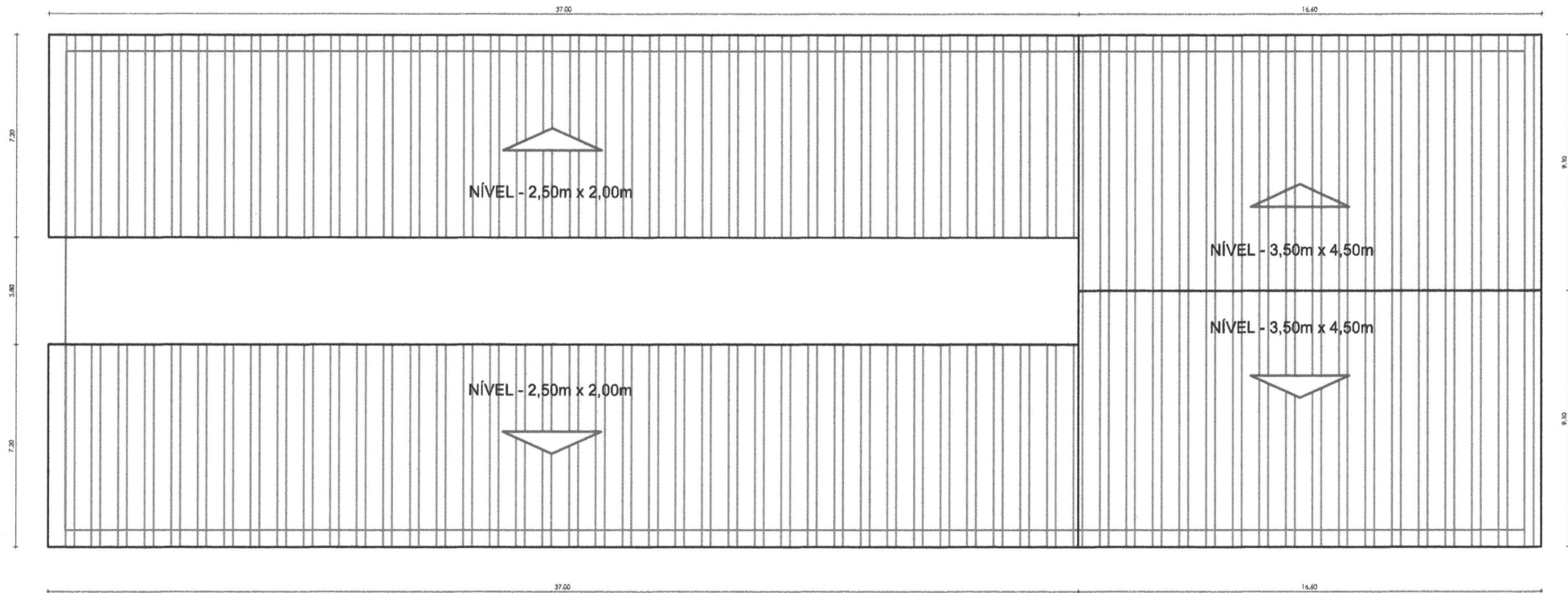
PLANTA DE COBERTURA Escala 1 : 100
