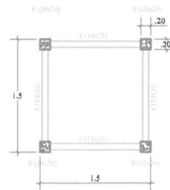
PLANTA BAIXA - NIVEL INTERMEDIÁRIO S/ESCALA
